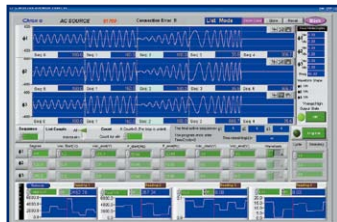
Optional Function LIST Mode Voltage Transient Output
